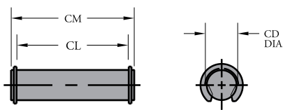
PIVOT PIN
