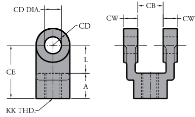
ROD CLEVIS
